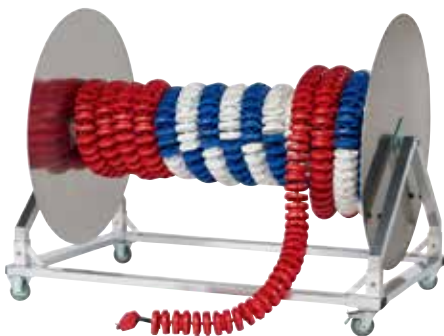
H088 - Enrouleur luxe mini Conçu pour 3 lignes d'eau Ø 150 mm de 50 m ou 6 lignes d'eau Ø 100 mm de 25 m 178 x 118 x 137 cm 2010,00 € HT
