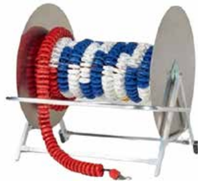
H087 - Enrouleur standard maxi Conçu pour 4 lignes Ø 100 de 25 m 140 x 135 x 139 cm 1899,00 € HT
